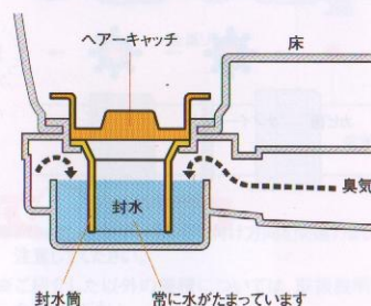
*排水トラップ断面図
